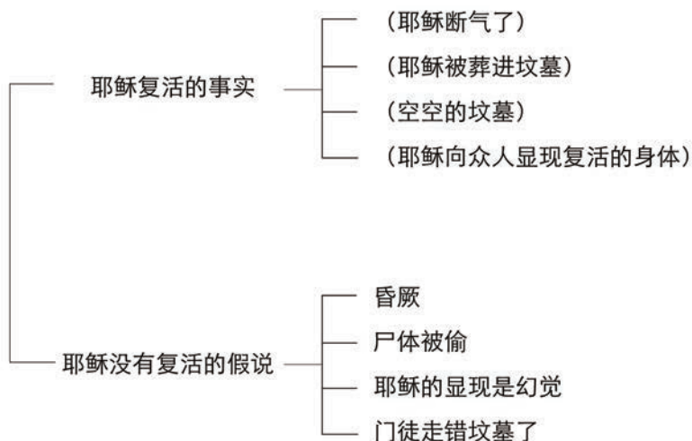
二分法图表
